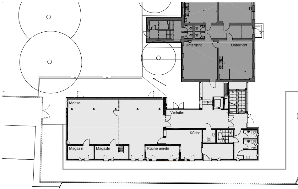
Buntentorsteinweg Grundschule, Bremen - Grundriss Erdgeschoss
