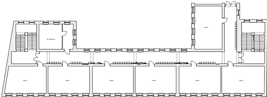
Erika-Mann-Grundschule, Berlin - Grundriss 2. Obergeschoss Entwurfsverfasser: Baupiloten, Berlin
