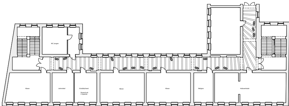
Erika-Mann-Grundschule, Berlin - Grundriss 1. Obergeschoss Entwurfsverfasser: Baupiloten, Berlin
